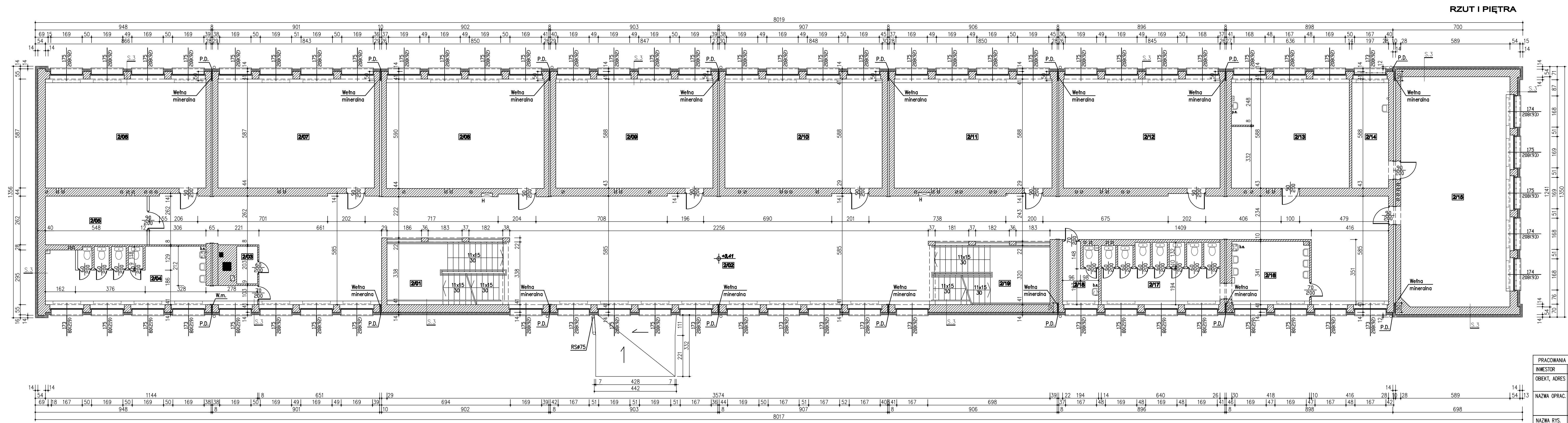
RZUT I PIĘTRA
